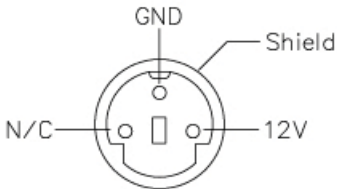
Mini-DIN 3P
